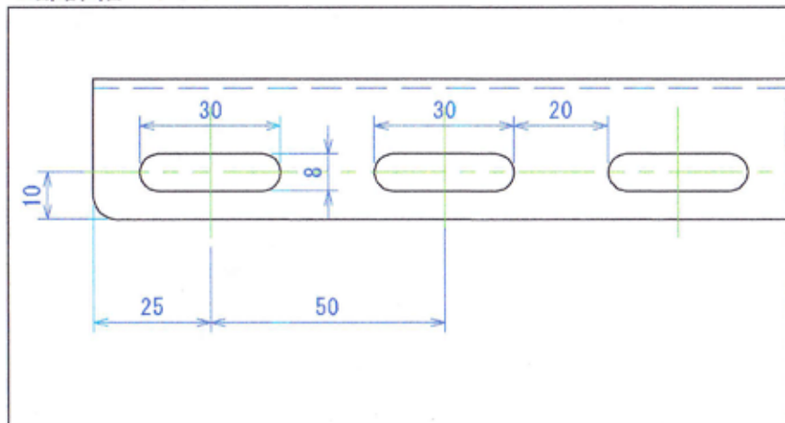
A部詳細 1:1
