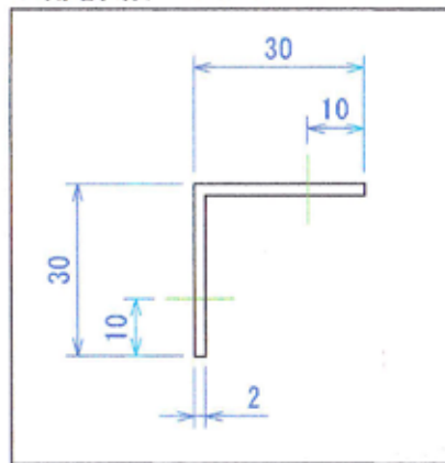
B部詳細 1:1
